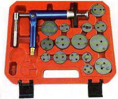
0065868 ARRETRATORE PISTONCINI FRENI CON ARRETRATORE PNEUMATICO
